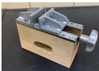
Étau de marque CI G4 Technique de soudage
